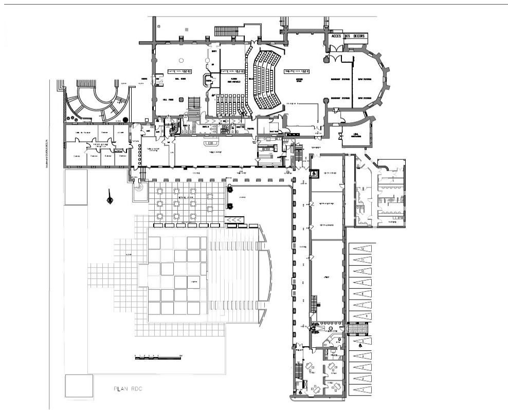
Rez-de-chaussée
